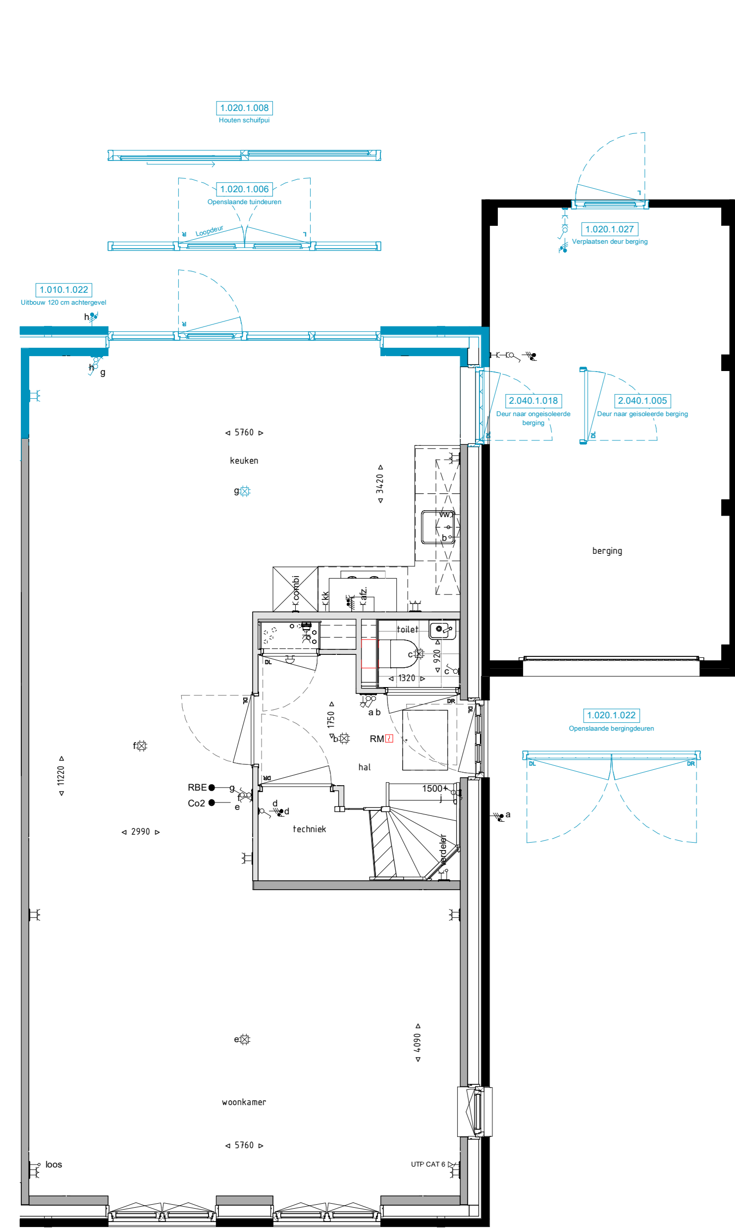
Begane grond 1 : 50
