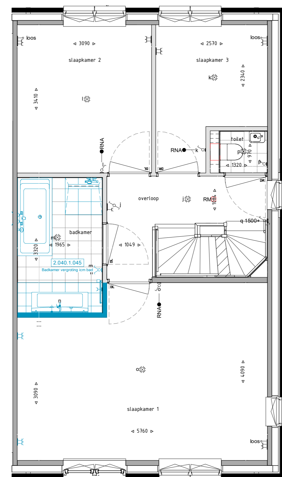
Eerste verdieping 1 : 50
