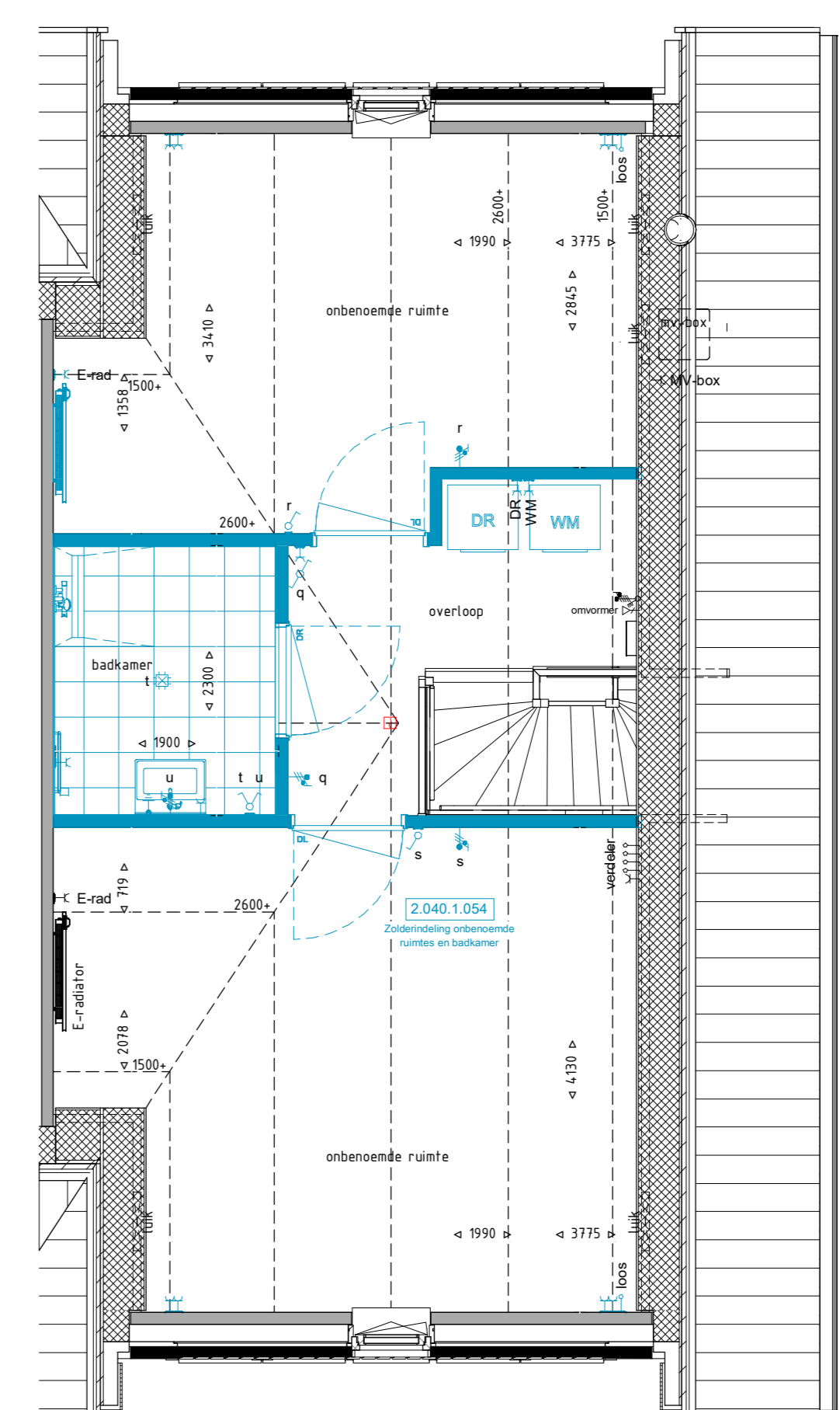
Tweede verdieping 1 : 50
