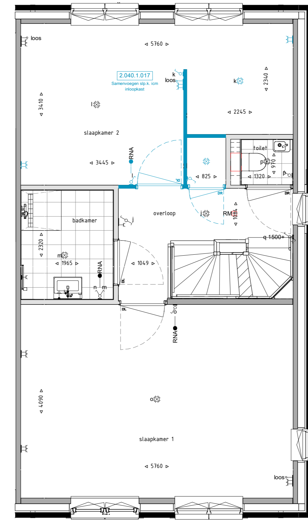
Eerste verdieping 1 : 50
