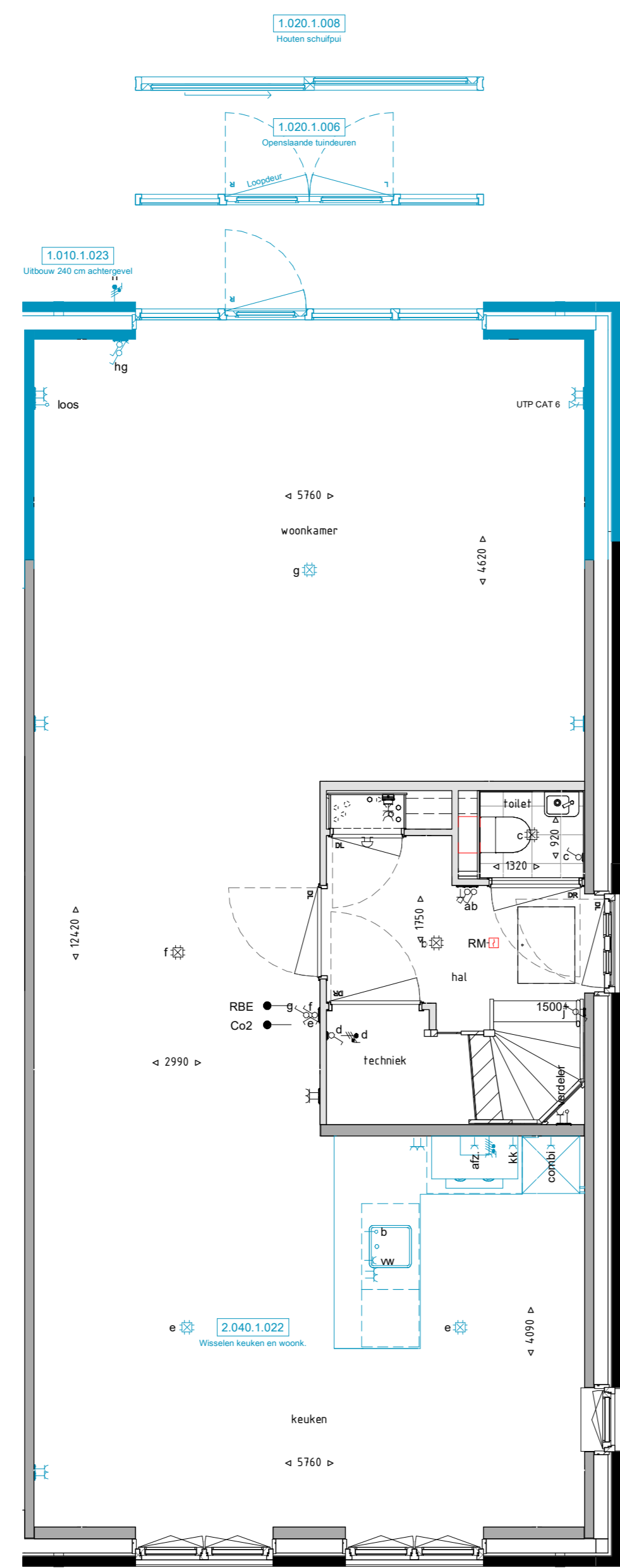
Begane grond 1 : 50
