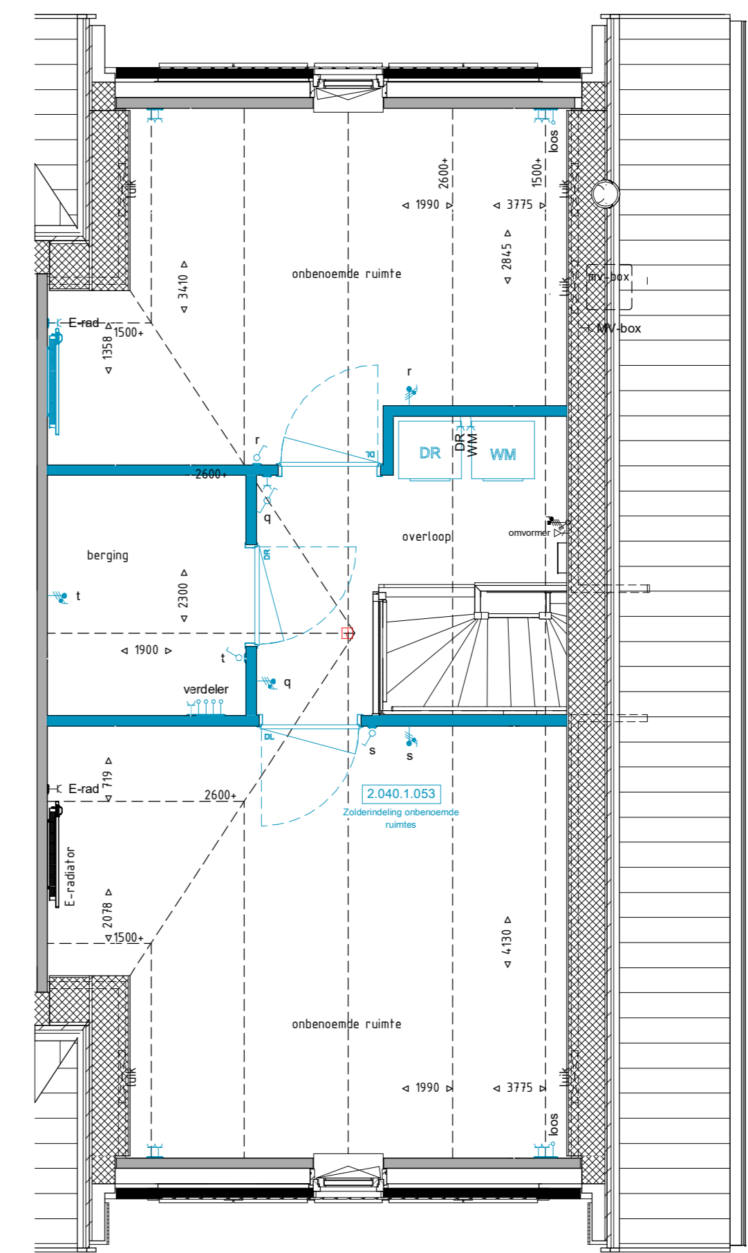
Tweede verdieping 1 : 50
