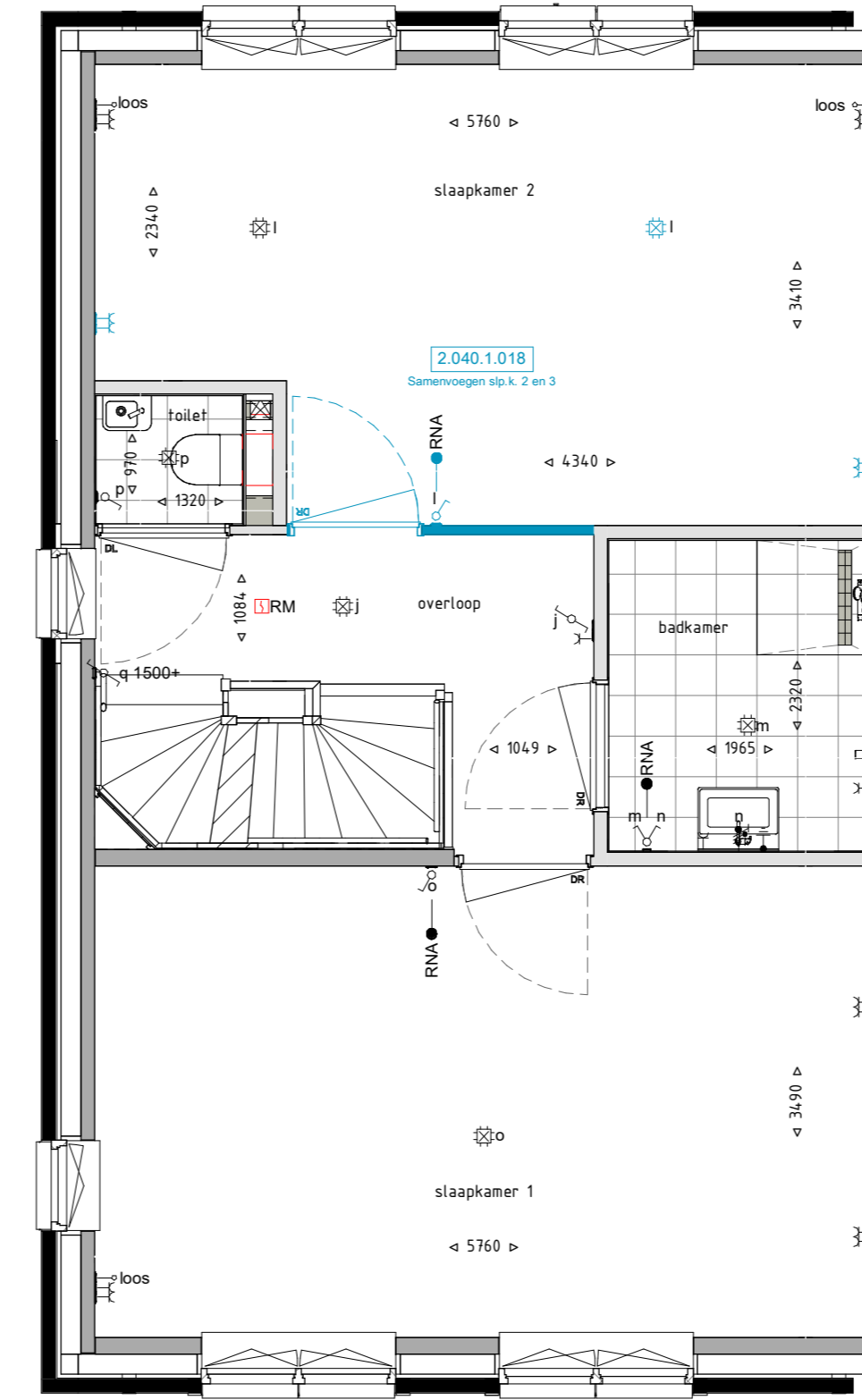
Eerste verdieping 1: 50
