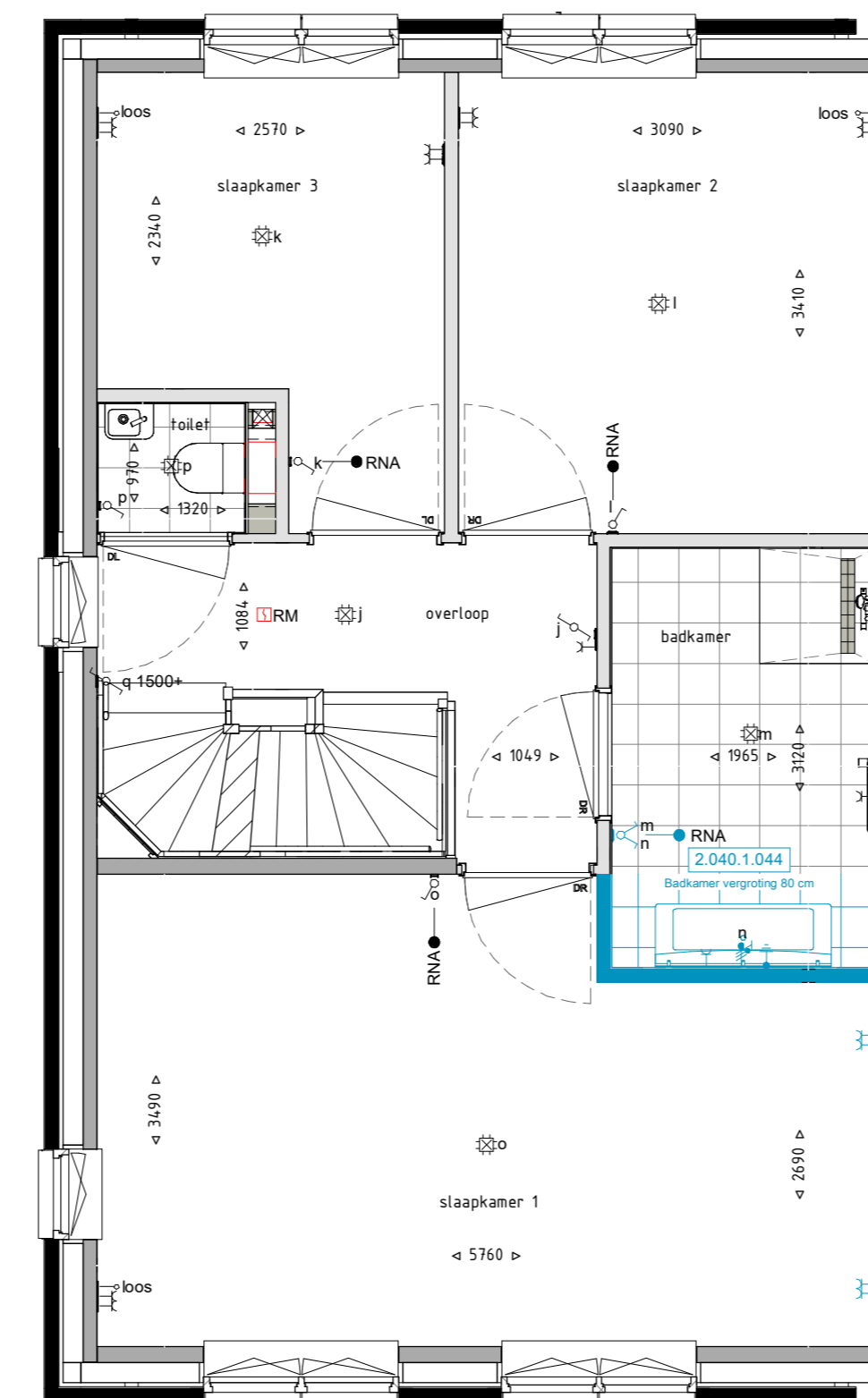
Eerste verdieping 1: 50
