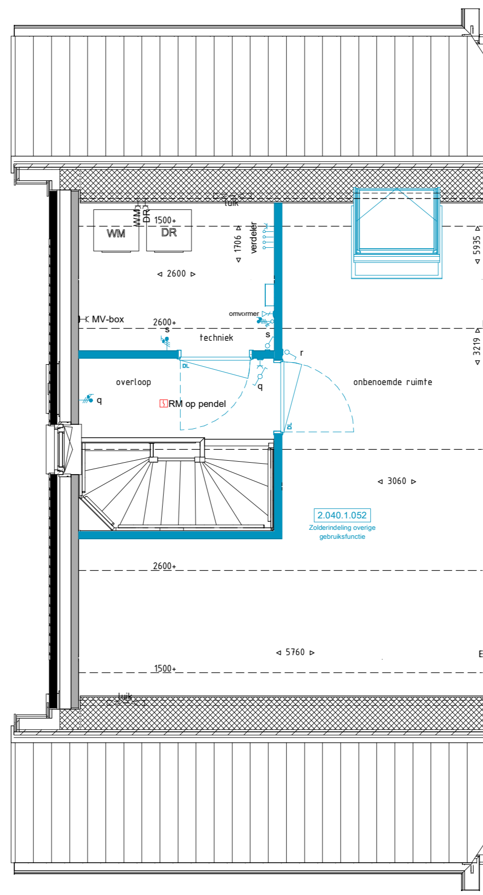
Tweede verdieping 1: 50
