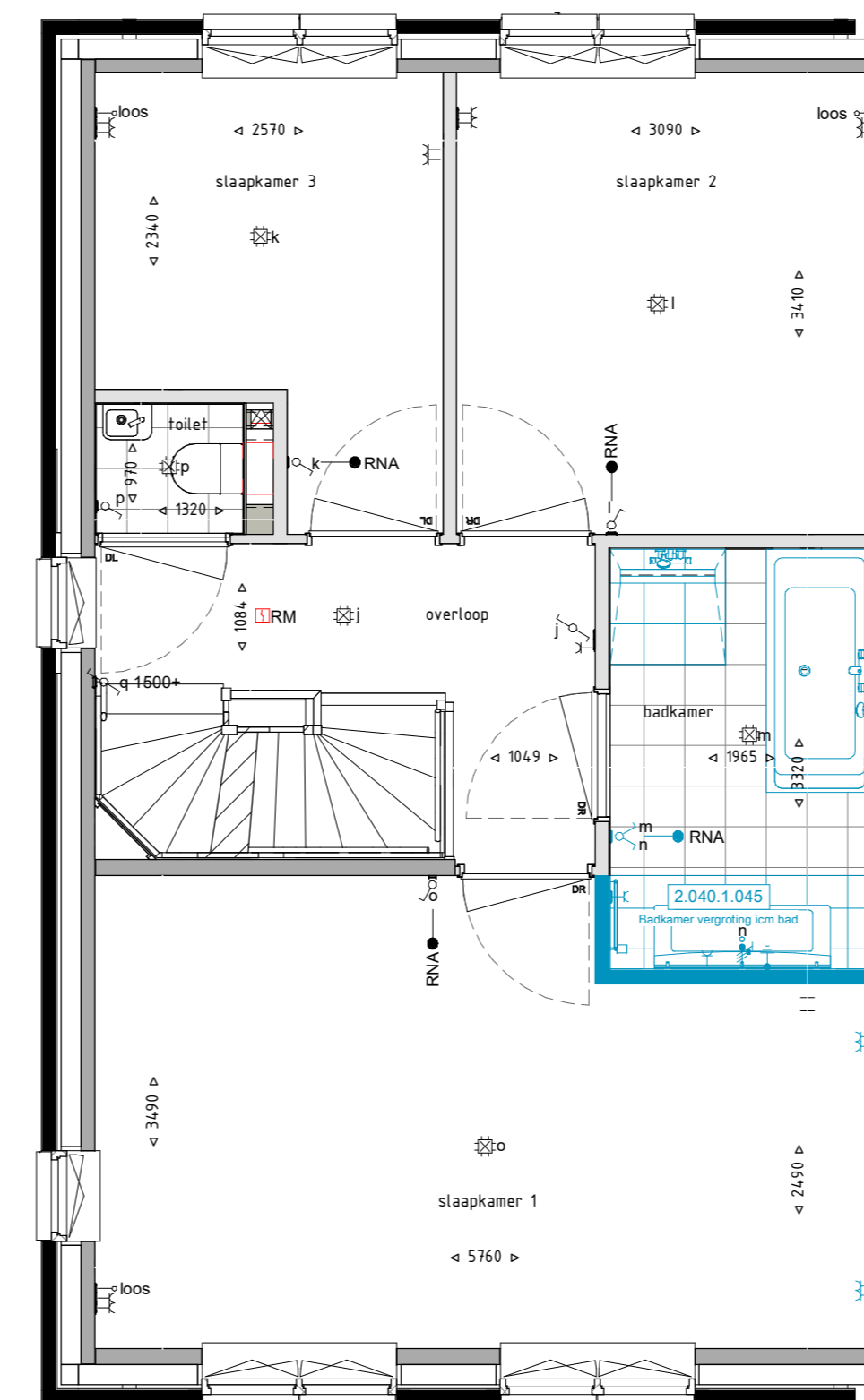
Eerste verdieping 1: 50
