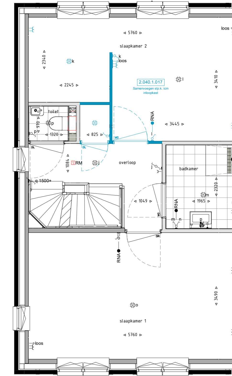
Eerste verdieping 1: 50
