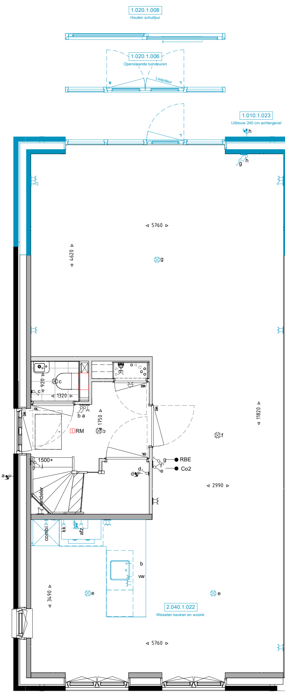
Eerste verdieping 1: 50
