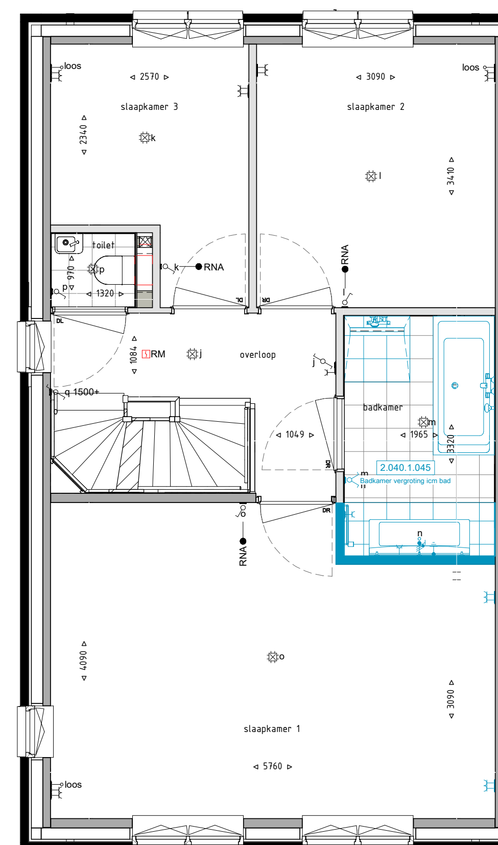
Eerste verdieping 1 : 50
