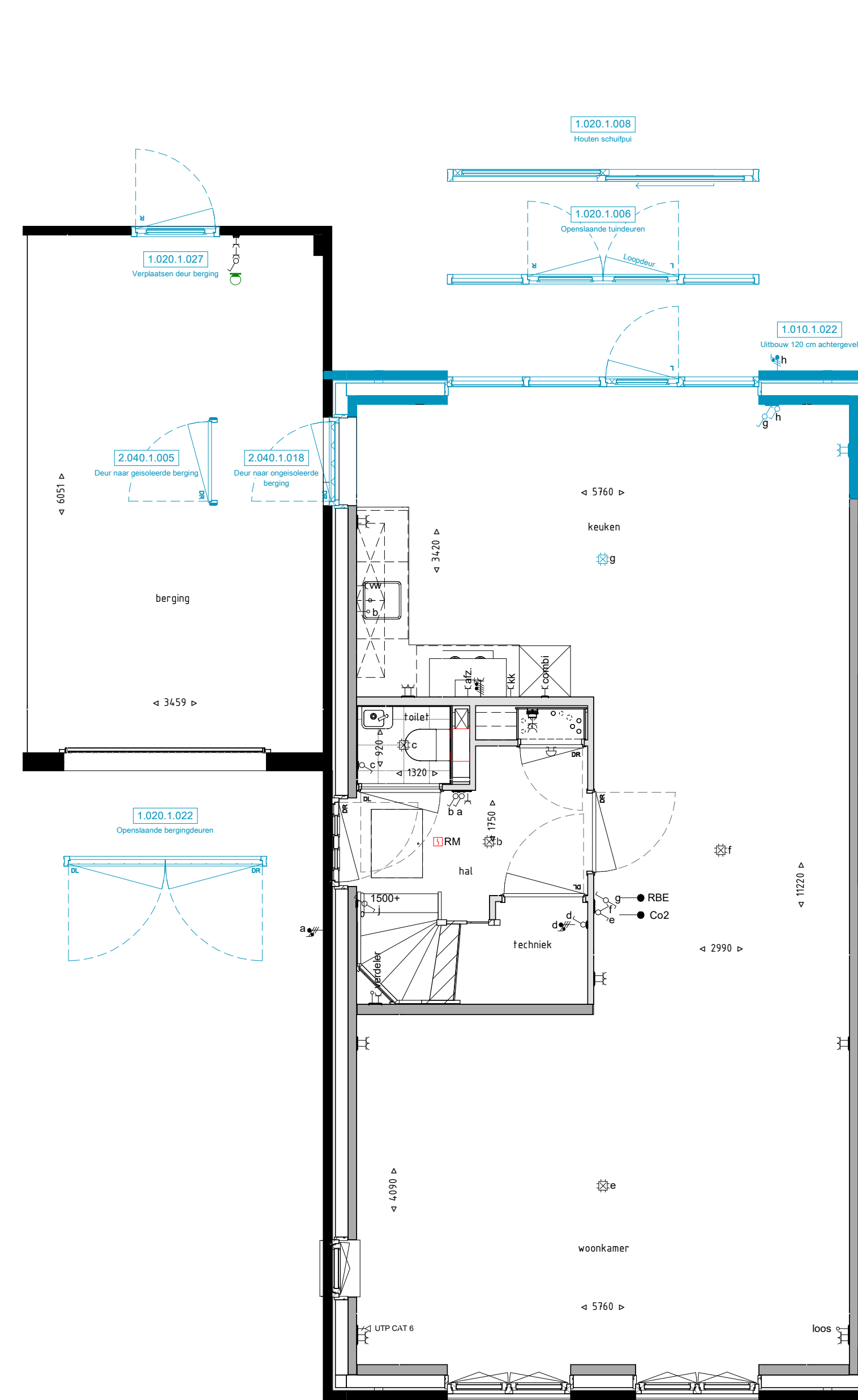
Begane grond 1 : 50
