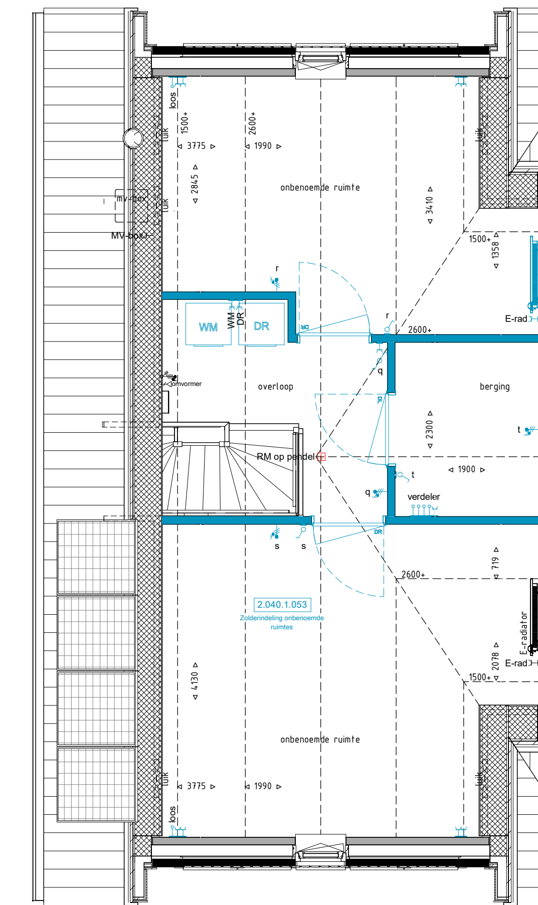
Tweede verdieping 1 : 50
