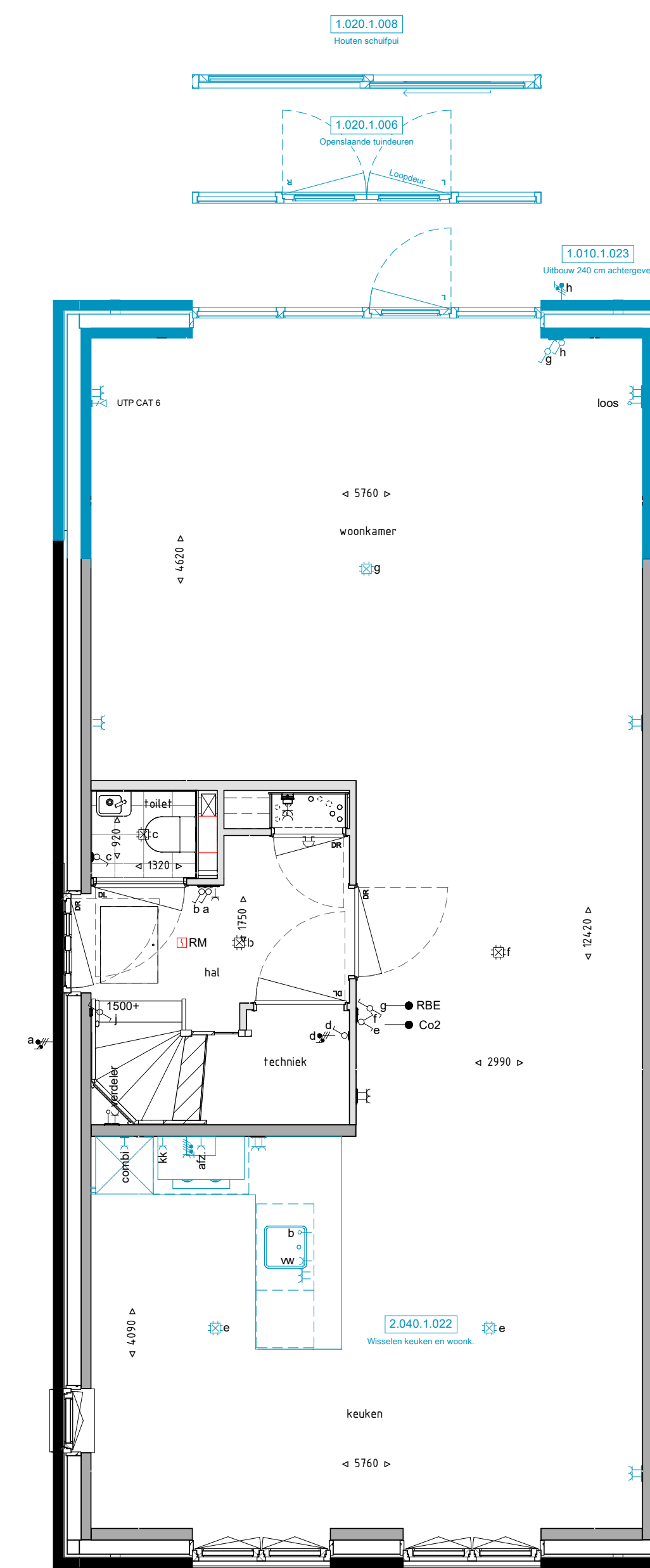
Begane grond 1 : 50
