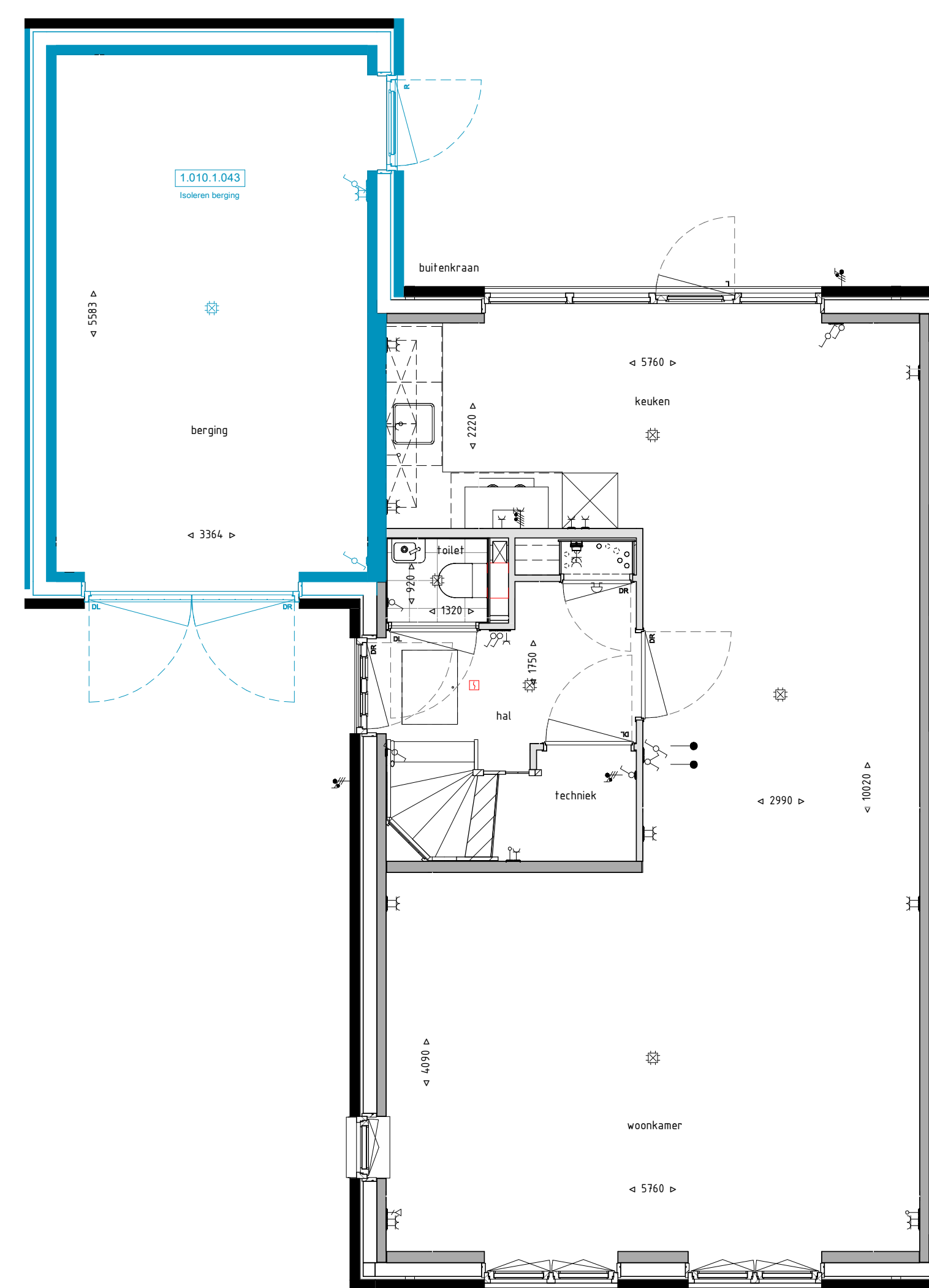
Begane grond 1 : 50
