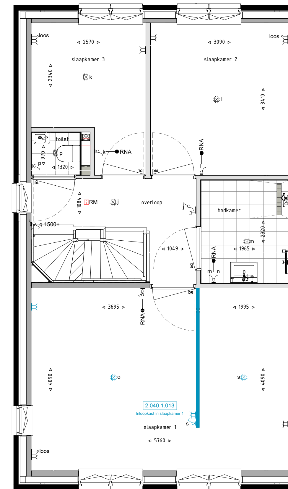
Eerste verdieping 1 : 50
